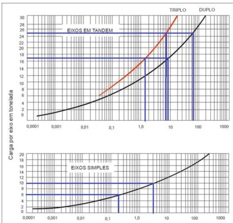
Gráfico 01 -Fator Equivalente de Operação – DNER.
